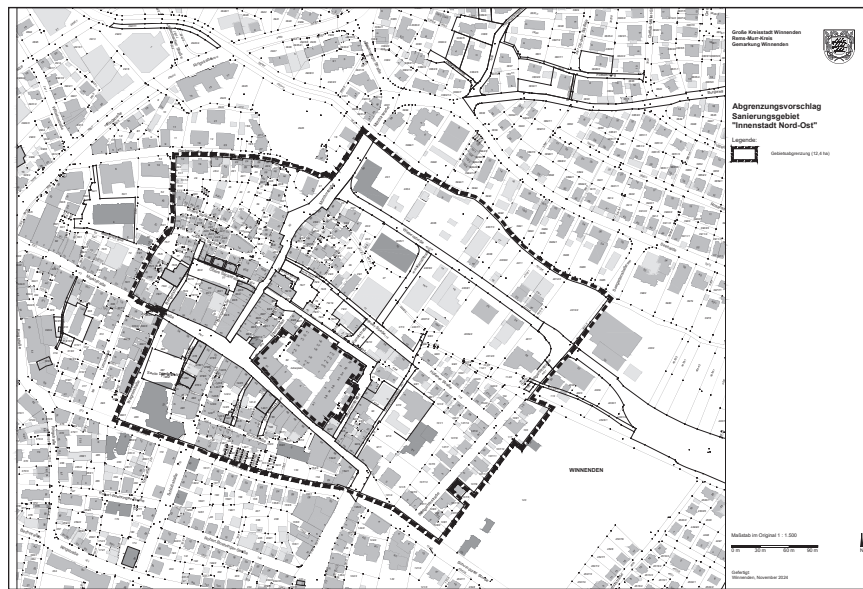
Lageplan November 2024.
